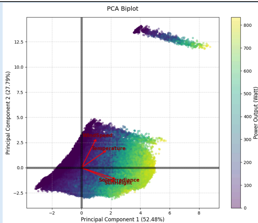
Gambar 8. Biplot PCA
